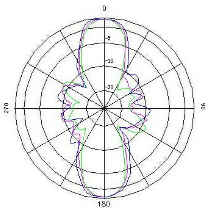
垂直面方向图 (2400)
