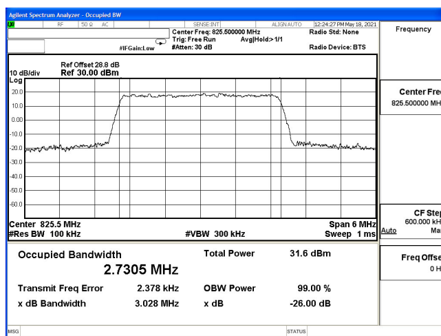
OCC-B5 3M-CH20415-QPSK
