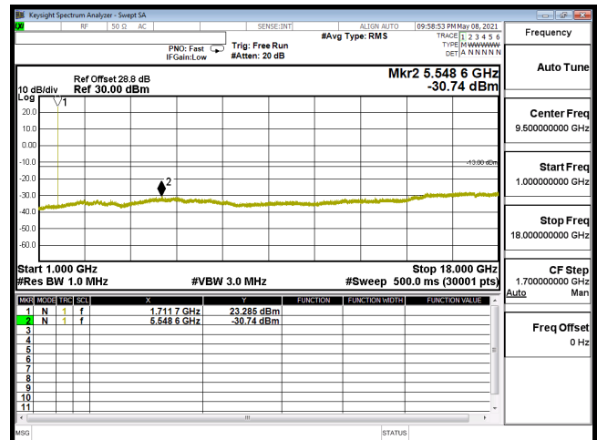
CSE-B66_3M-CH131987-QPSK(1,7)-1G-18G
