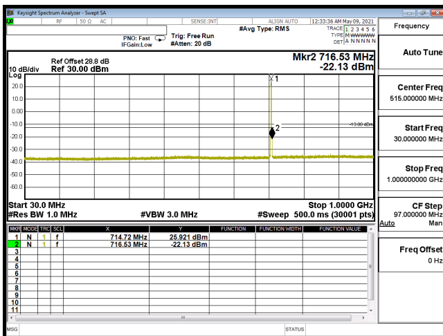
CSE-B12_3M-CH23165-16QAM(1,7)-30M-1G
