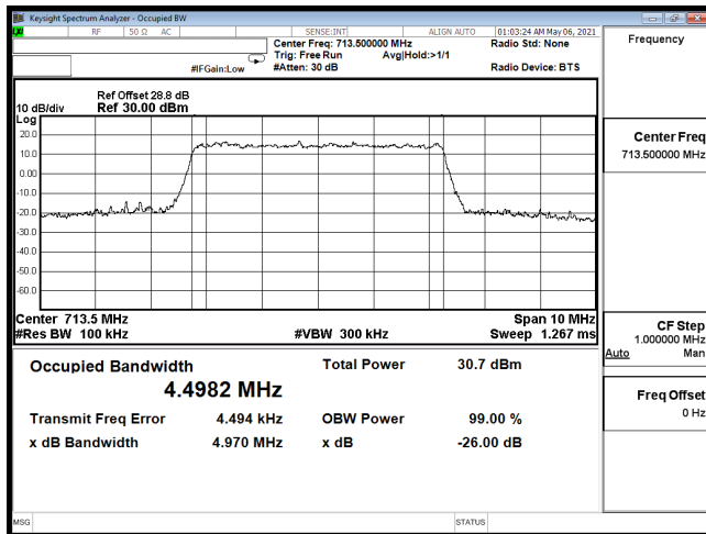
OCC-B12_5M-CH23155-QPSK
