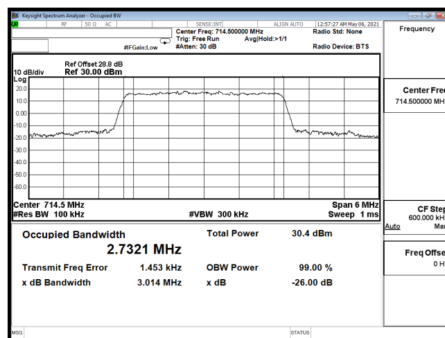
OCC-B12_3M-CH23165-QPSK
