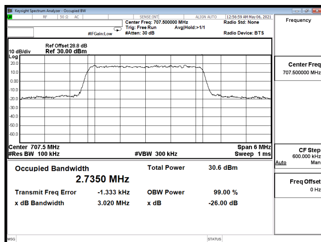
OCC-B12_3M-CH23095-QPSK
