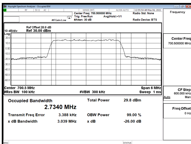
OCC-B12_3M-CH23017-16QAM
