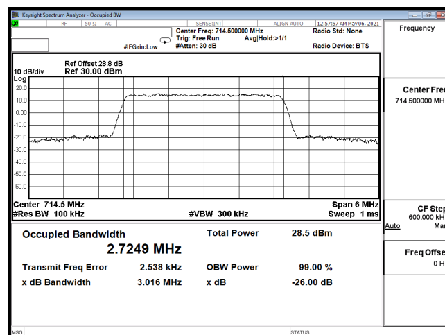
OCC-B12_3M-CH23165-64QAM
