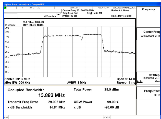
OCC(10M+5M)-2ULCA_5B-QPSK_829(50,0)+836.2(25,0)
