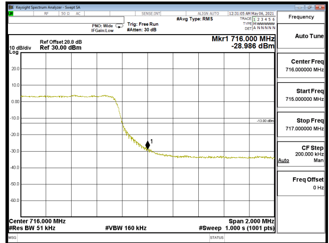
EDGE-B12_5M-CH23155-QPSK(25,0)
