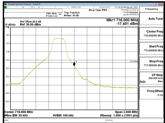
EDGE-B12_3M-CH23165-QPSK(1,14)
