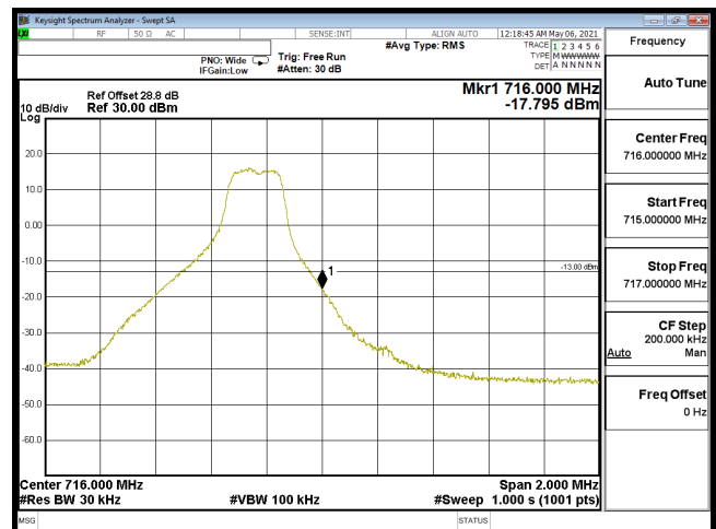
EDGE-B12_3M-CH23165-16QAM(1,14)
