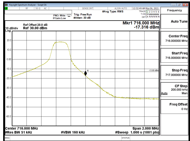
EDGE-B12_5M-CH23155-QPSK(1,24)
