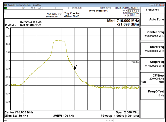
EDGE-B12_3M-CH23165-64QAM(1,14)
