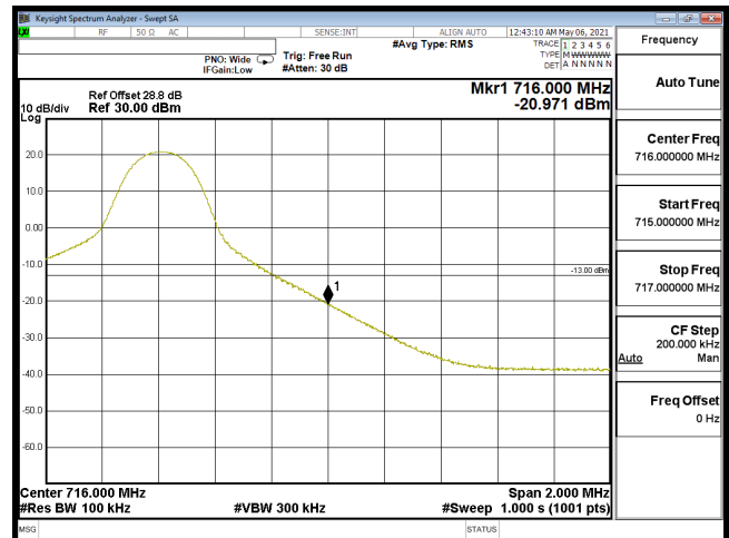
EDGE-B12_10M-CH23130-QPSK(1,49)
