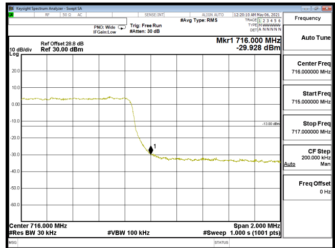
EDGE-B12_3M-CH23165-QPSK(15,0)
