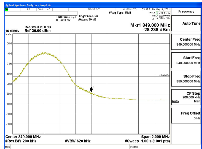
EDGE(10M+10M)-2ULCA_5B-QPSK_834.1(1,0)+844(1,49)
