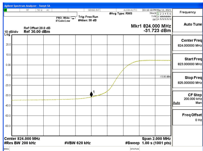
EDGE(10M+10M)-2ULCA_5B-QPSK_829(50,0)+838.9(50,0)
