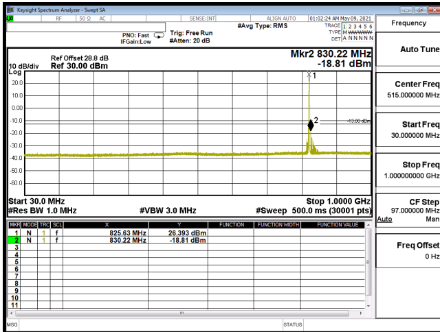
CSE-B5_3M-CH20415-QPSK(1,7)-30M-1G
