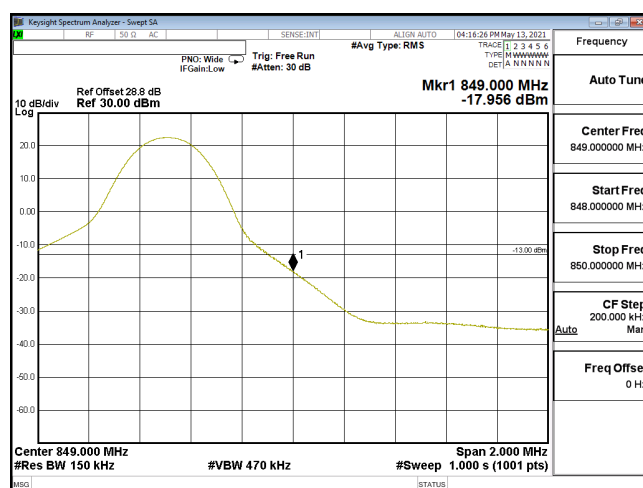
EDGE-ENDC 30A n5-QPSK 15M CH168300 841.5(1,78) SCS15KHz
