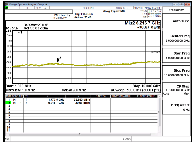
CSE-B66_5M-CH132647-QPSK(1,12)-1G-18G
