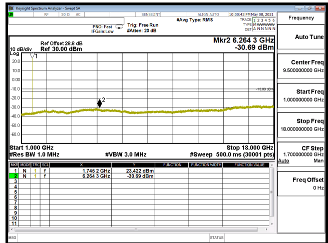
CSE-B66_3M-CH132322-QPSK(1,7)-1G-18G
