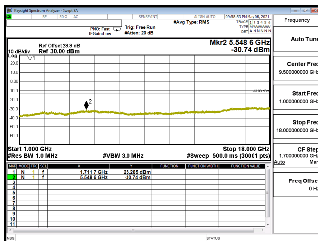
CSE-B66_3M-CH131987-QPSK(1,7)-1G-18G
