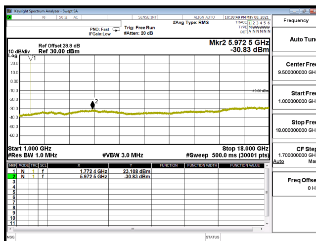
CSE-B66_15M-CH132597-16QAM(1,37)-1G-18G
