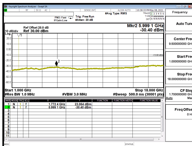
CSE-B66_15M-CH132597-QPSK(1,37)-1G-18G
