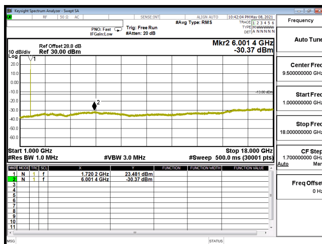
CSE-B66_20M-CH132072-QPSK(1,50)-1G-18G
