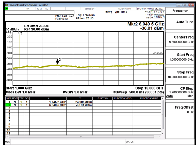
CSE-B66_15M-CH132322-QPSK(1,37)-1G-18G
