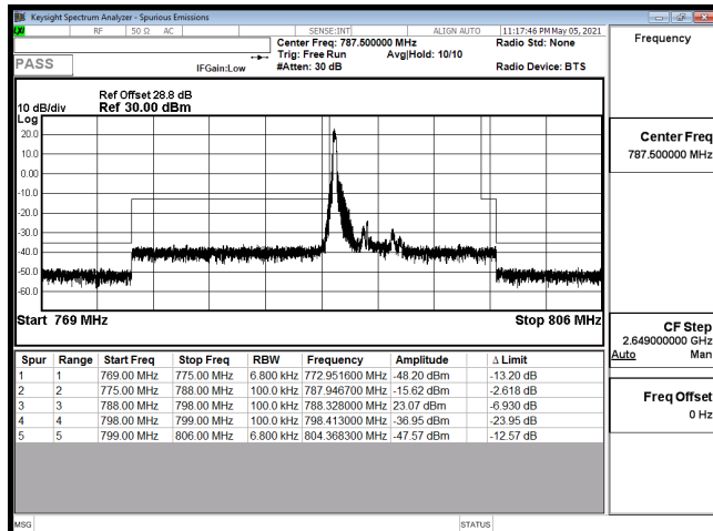
EDGE-B14 5M-CH23305-QPSK(1,0)
