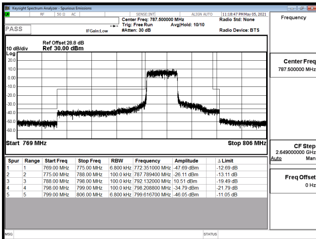
EDGE-B14 5M-CH23305-QPSK(25,0)
