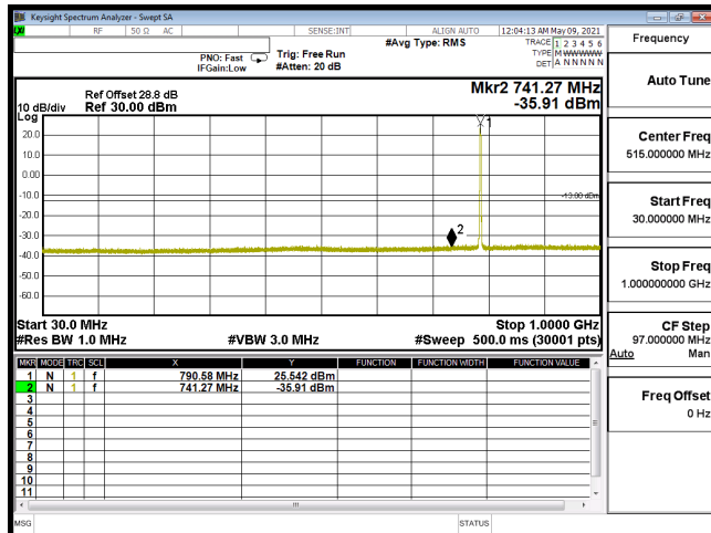
CSE-B14 5M-CH23305-QPSK(1,12)-30M-1G
