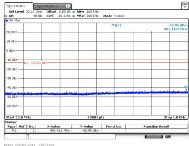
WCDMA_B4_CH1413_RMC_under 1G
