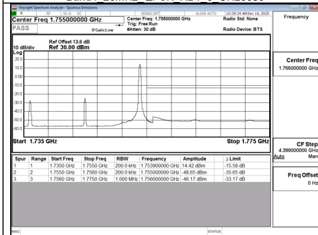
Band4 20MHz QPSK RB1 99 CH20300
