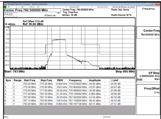
Band13 5MHz QPSK RB25 0 CH23205
