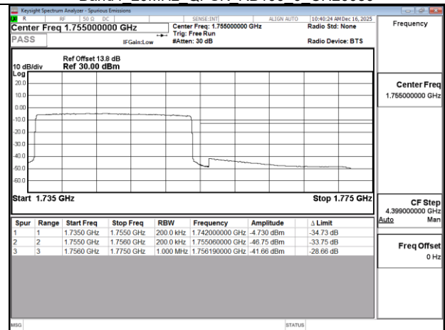
Band4 20MHz QPSK RB100 0 CH20300
