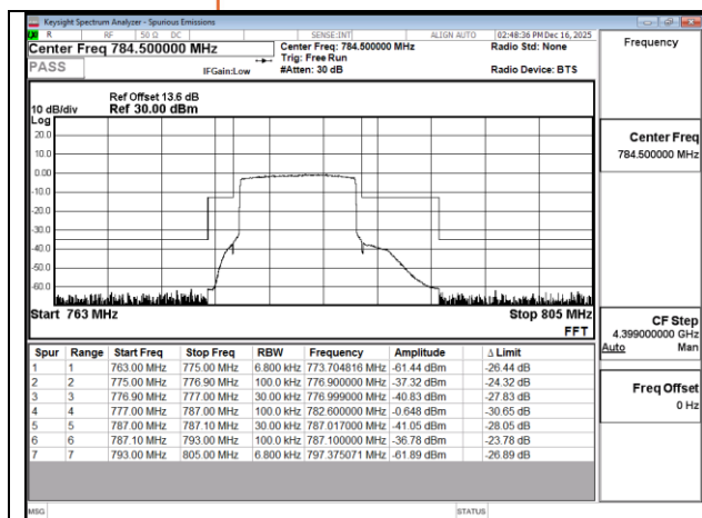
Band13_10MHz_QPSK_RB50_0_CH23230
