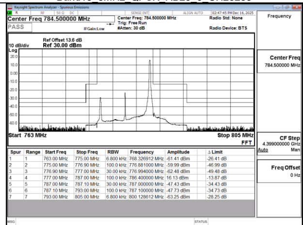
Band13 10MHz QPSK RB1 49 CH23230
