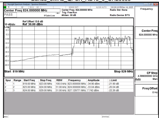
Band5 5MHz QPSK RB25 0 CH20425
