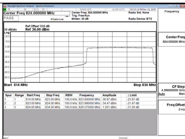
Band5 10MHz QPSK RB50 0 CH20450
