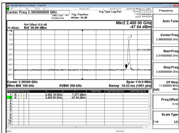
Band Edge GFSK 1M DH5 2402MHz
