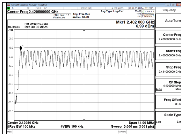
GFSK 1M DH5 2400-2441
