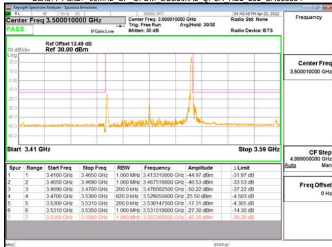
Band77-Part27 60MHz CP OFDM SCS30kHz QPSK RB1 161 CH634666
