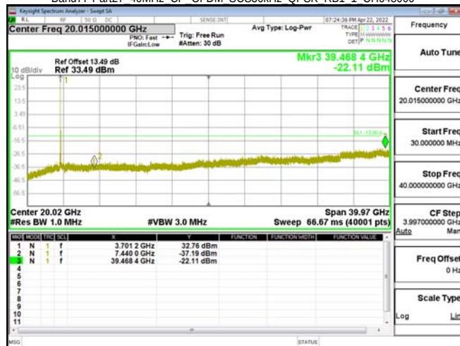
Band77-Part27 40MHz CP OFDM SCS30kHz QPSK RB1 1 CH656000
