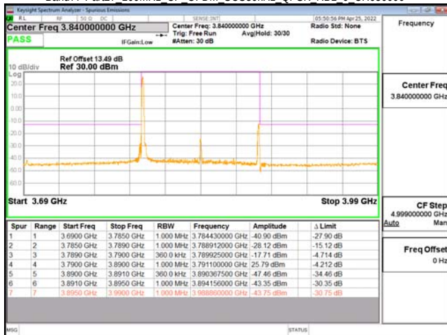
Band77-Part27 100MHz CP OFDM SCS30kHz QPSK RB1 0 CH656000
