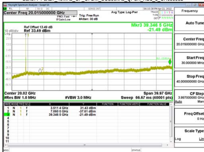
Band77-Part27 40MHz CP OFDM SCS30kHz QPSK RB1 1 CH635332
