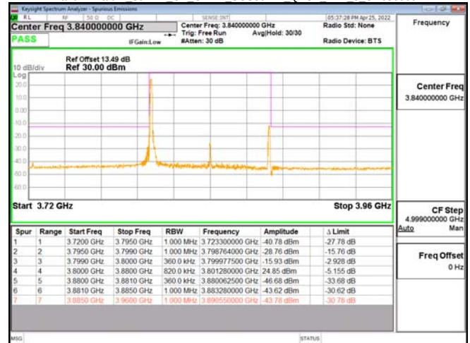
Band77-Part27 80MHz CP OFDM SCS30kHz QPSK RB1 0 CH662666
