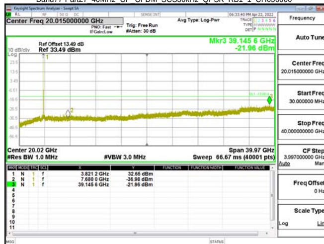
Band77-Part27 40MHz CP OFDM SCS30kHz QPSK RB1 1 CH664000
