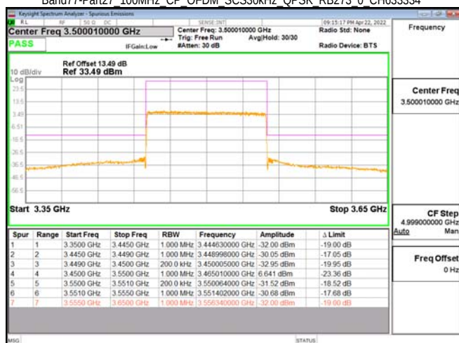
Band77-Part27 100MHz CP OFDM SCS30kHz QPSK RB273 0 CH633334
