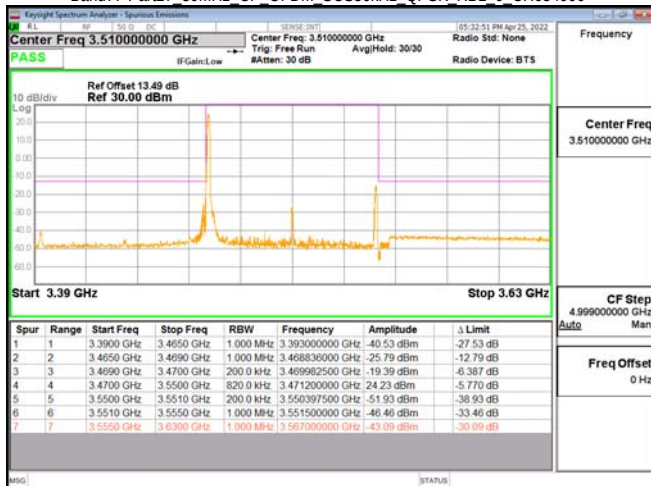
Band77-Part27 80MHz CP OFDM SCS30kHz QPSK RB1 0 CH634000
