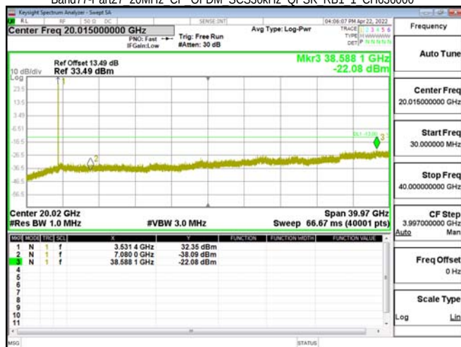
Band77-Part27_20MHz_CP_OFDM_SCS30kHz_QPSK_RB1_1_CH636000
