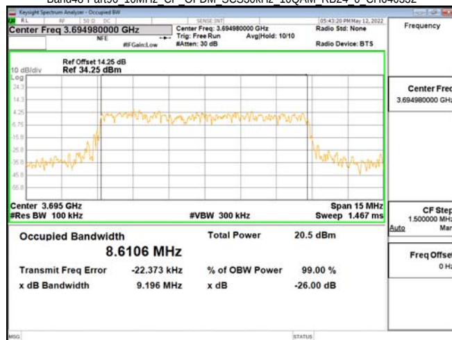
Band48-Part96 10MHz CP OFDM SCS30kHz 16QAM RB24 0 CH646332
