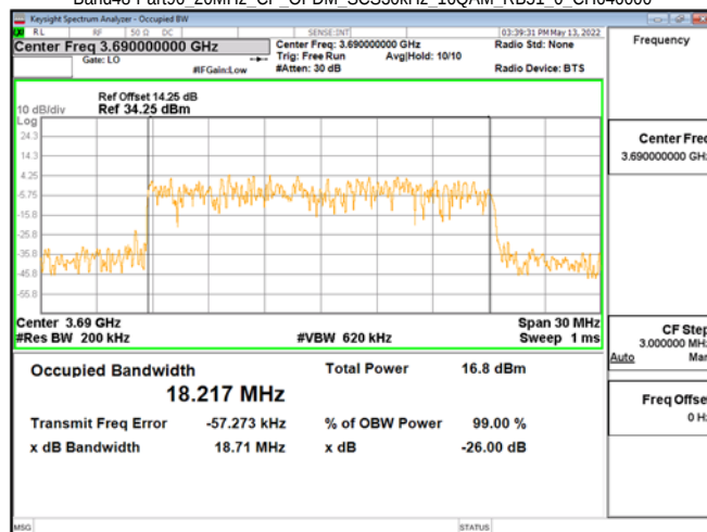
Band48-Part96 20MHz CP OFDM SCS30kHz 16QAM RB51 0 CH646000
