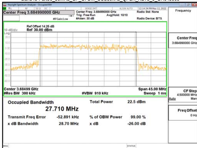
Band48-Part96 30MHz CP OFDM SCS30kHz QPSK RB78 0 CH645666
