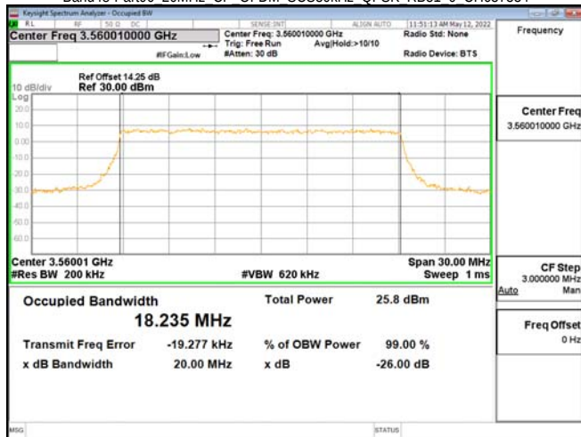
Band48-Part96 20MHz CP OFDM SCS30kHz QPSK RB51 0 CH641666
