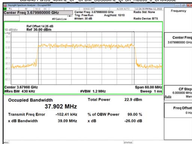
Band48-Part96 40MHz CP OFDM SCS30kHz QPSK RB106 0 CH645332
