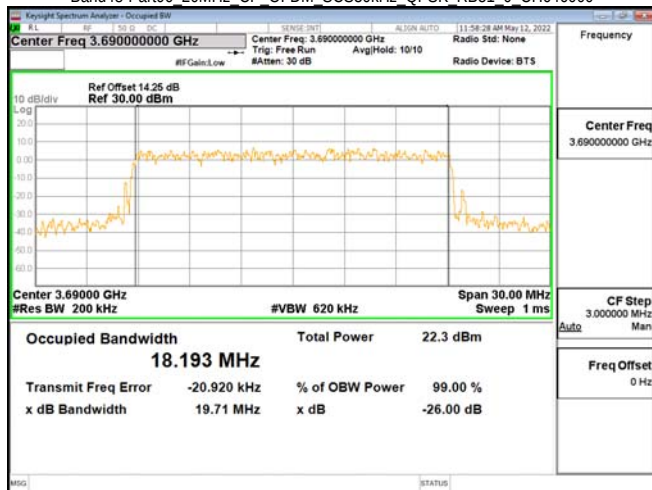
Band48-Part96 20MHz CP OFDM SCS30kHz QPSK RB51 0 CH646000
