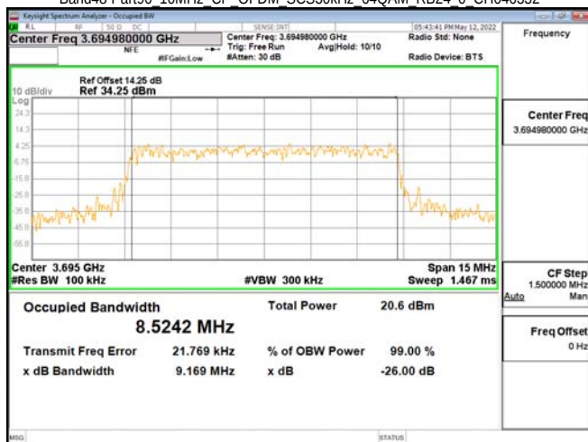
Band48-Part96 10MHz CP OFDM SCS30kHz 64QAM RB24 0 CH646332
