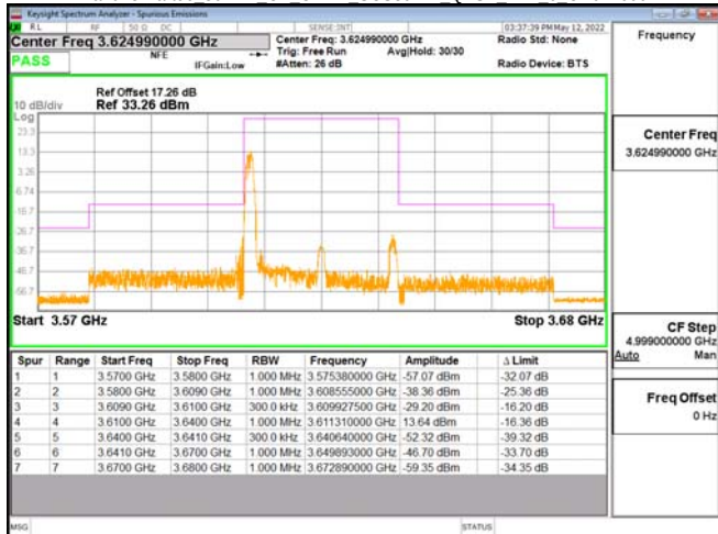
Band48-Part96 30MHz CP OFDM SCS30kHz QPSK RB1 0 CH645666
