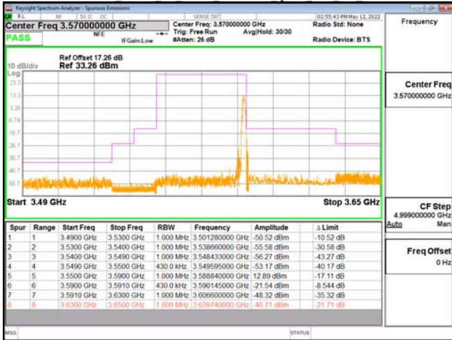
Band48-Part96 40MHz CP OFDM SCS30kHz QPSK RB1 105 CH641666
