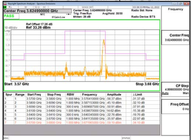
Band48-Part96 30MHz CP OFDM SCS30kHz QPSK RB1 77 CH645666
