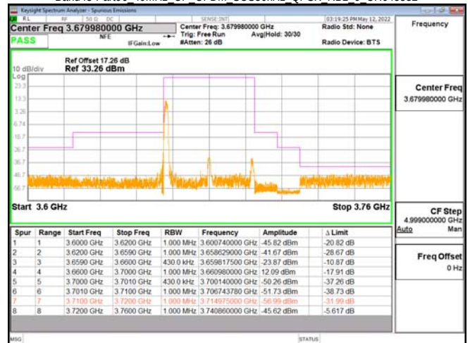
Band48-Part96 40MHz CP OFDM SCS30kHz QPSK RB1 0 CH645332
