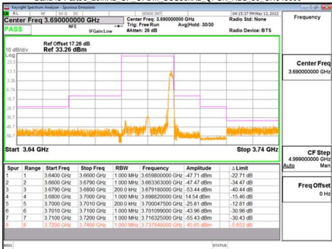
Band48-Part96 20MHz CP OFDM SCS30kHz QPSK RB1 50 CH646000
