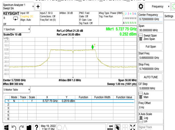
802.11ac_20MHz_Chain1_5720MHz_UNII 3
