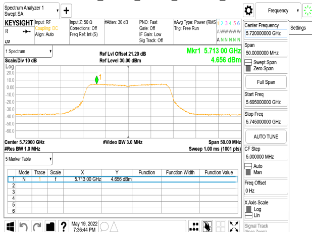
802.11ac_20MHz_Chain0_5720MHz_UNII 2C
