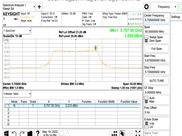
802.11a_20MHz_Chain3_5700MHz
