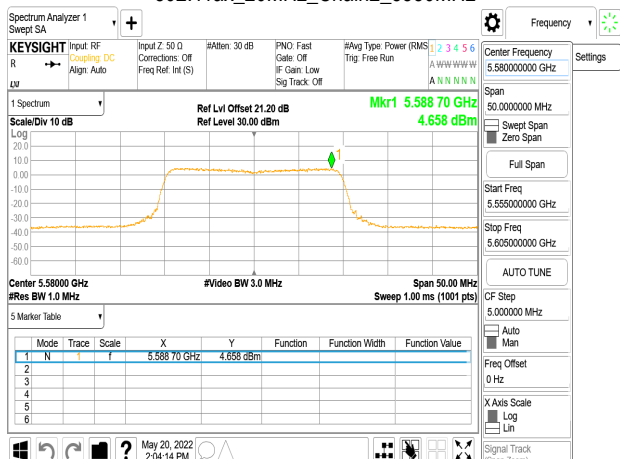
802.11ax_20MHz_Chain2_5580MHz
