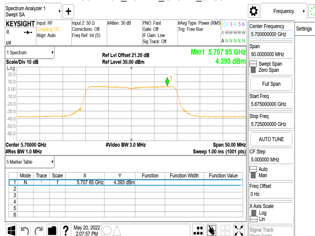
802.11ax_20MHz_Chain2_5700MHz_RU106_54
