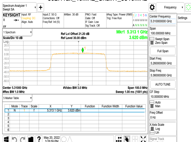
802.11ax_40MHz_Chain1_5310MHz_RU242_62
