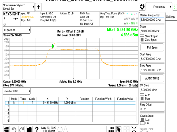
802.11ax_20MHz_Chain2_5500MHz_RU106_53
