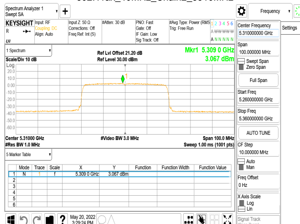
802.11ax_40MHz_Chain2_5310MHz
