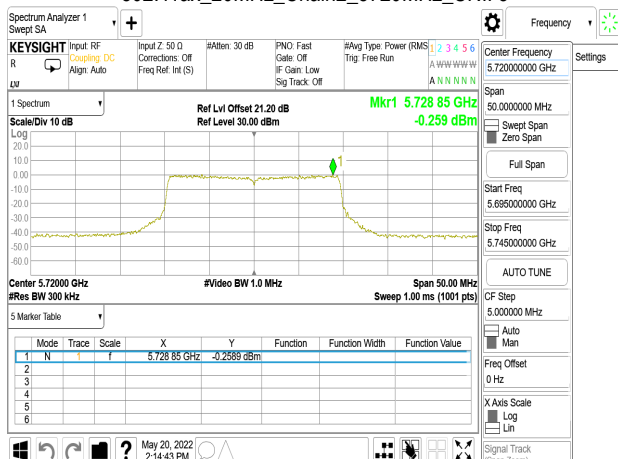
802.11ax_20MHz_Chain2_5720MHz_UNII 3
