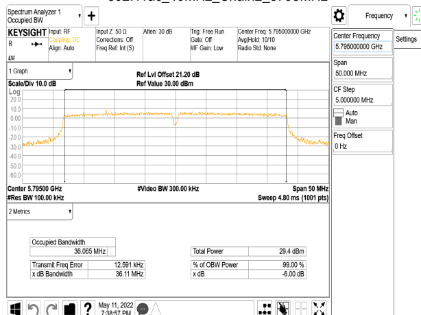
802.11ac 40MHz Chain2 5795MHz
