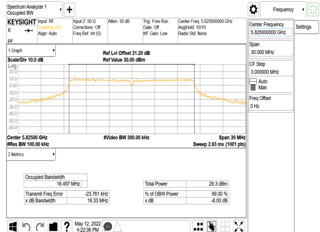
802.11a_20MHz_Chain2_5825MHz
