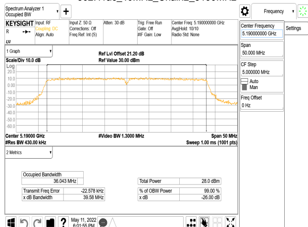
802.11ac 40MHz Chain2 5190MHz
