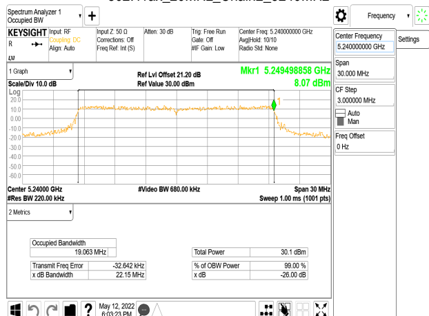
802.11ax_20MHz_Chain2_5240MHz
