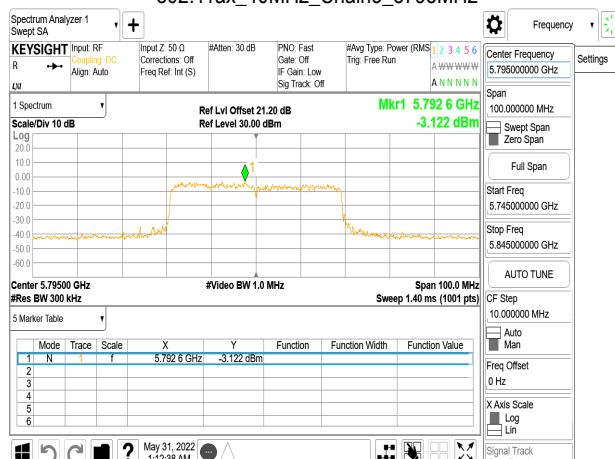
802.11ax_40MHz_Chain3_5795MHz_RU242_62
