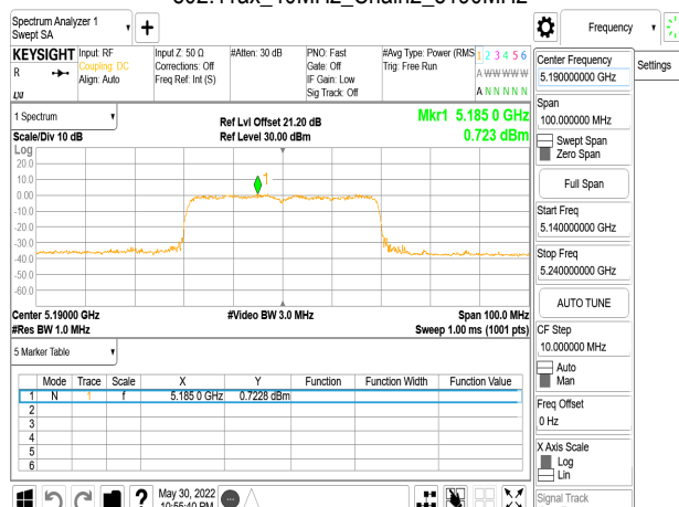
802.11ax_40MHz_Chain2_5190MHz_RU242_61
