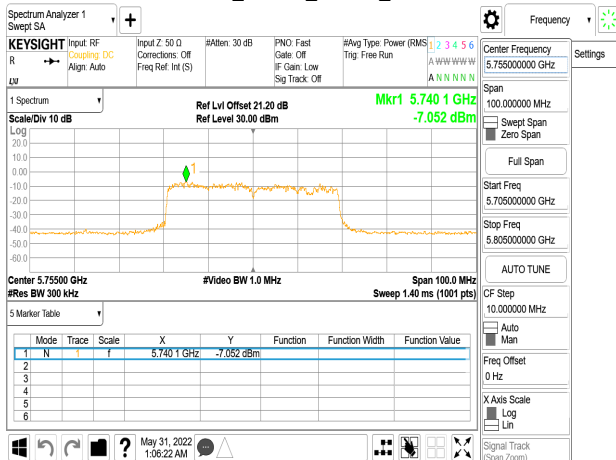
802.11ax_40MHz_Chain2_5755MHz_RU242_61
