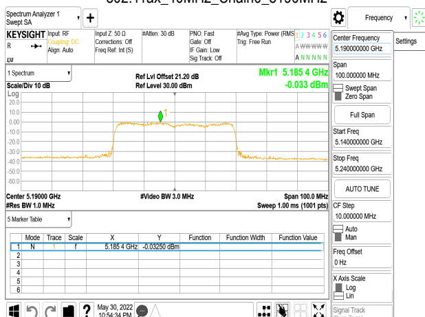
802.11ax_40MHz_Chain0_5190MHz_RU242_61
