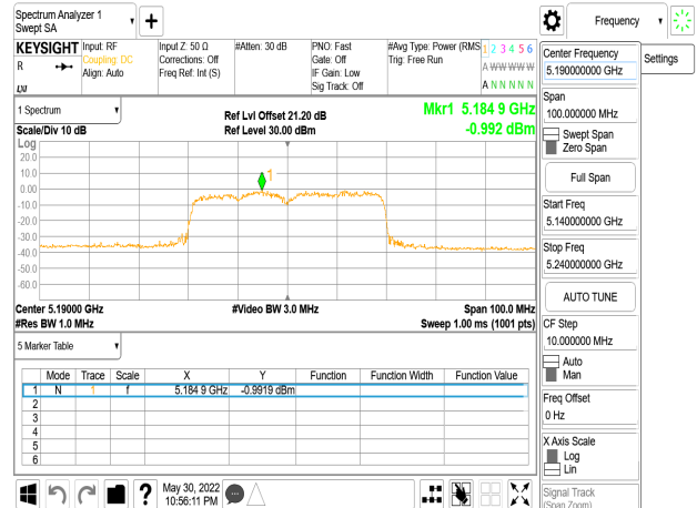
802.11ax_40MHz_Chain3_5190MHz_RU242_61
