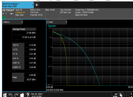
B2_N66(20M)_DFT-s-OFDM_PI_2-BPSK_Edge_1RB_Left_Low_CH
