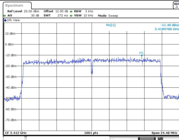
11AX20MIMO_Ant5_2412
