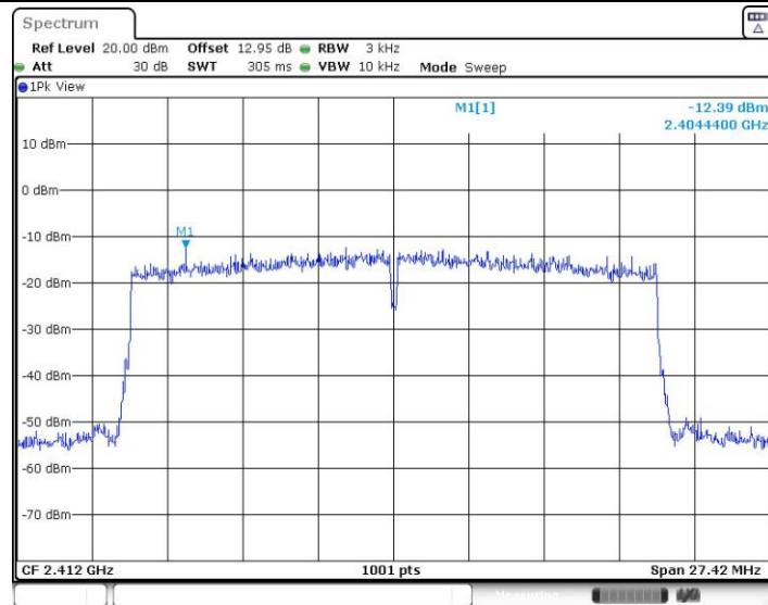
11AX20MIMO_Ant4_2412
