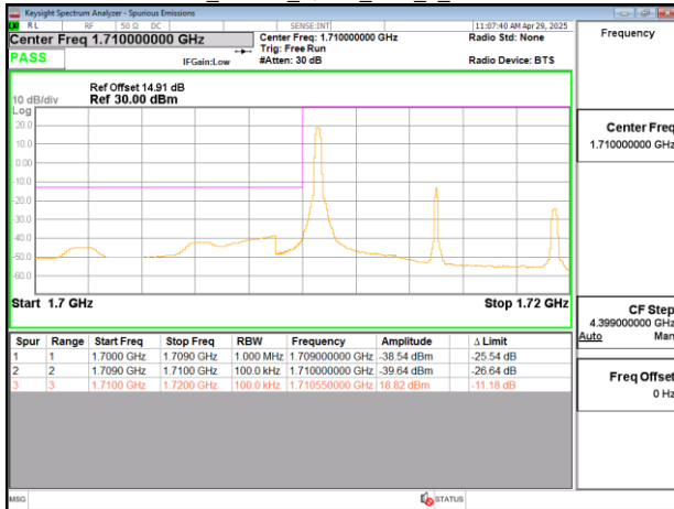
Band4_10MHz_QPSK_RB50_0_CH20000
