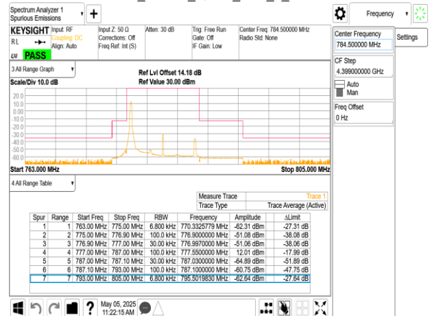
Band13_10MHz_QPSK_RB1_49_CH23230
