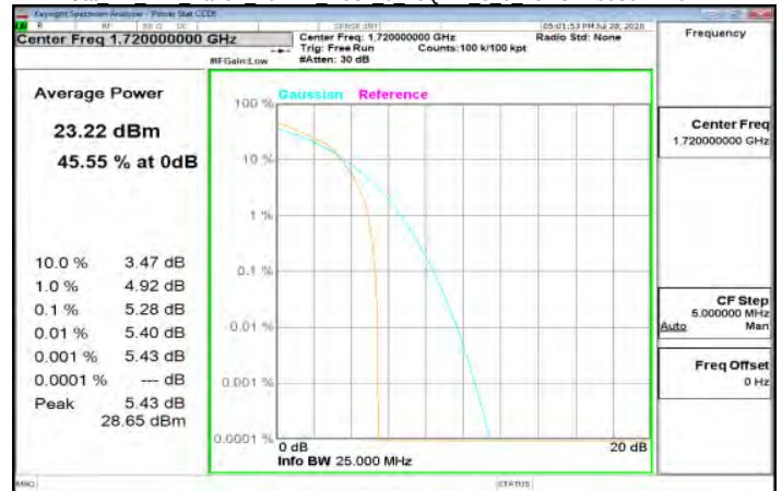
Cat M1 LTE Band4 20MHz index 0 16QAM 6 0 LowCH20050-1720
