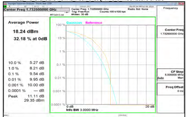
Cat M1 LTE Band4 3MHz index 0 16QAM 6 0 MidCH20175-1732.5
