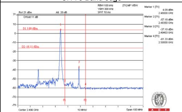
CH 78 Band edge
