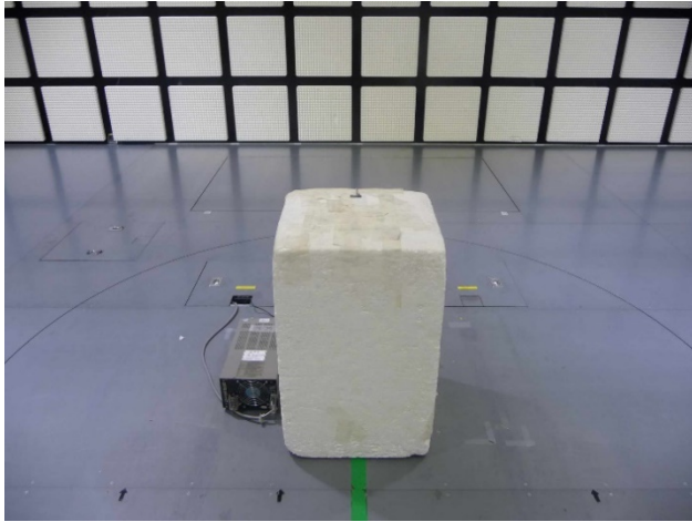
BT LE Front
