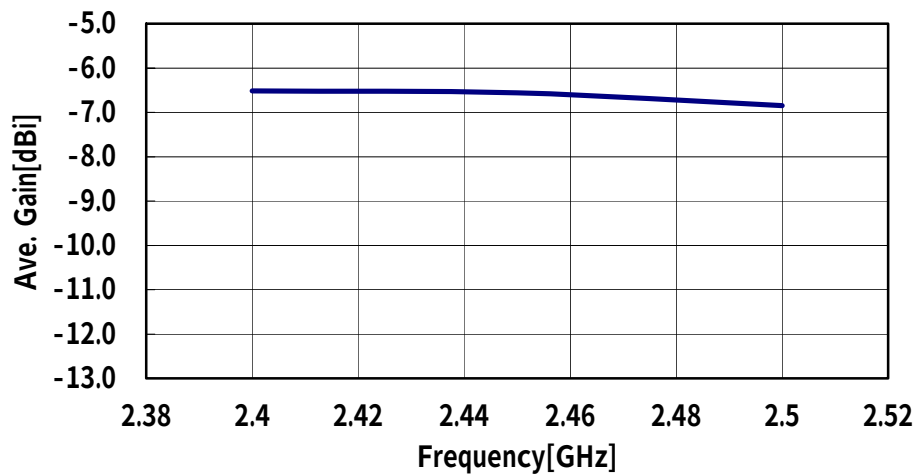
図16. 平均利得の周波数特性 (Bluetooth)
