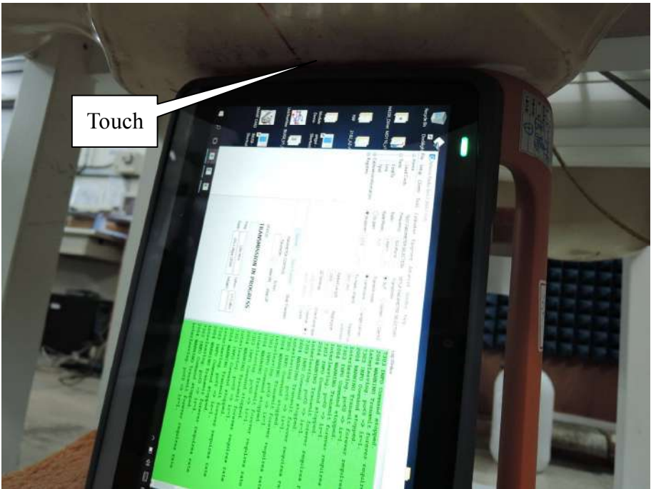
Left-Side (TX2)
