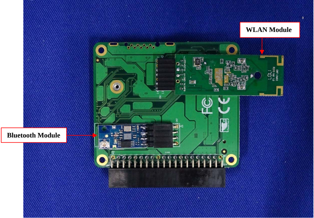
(12) EUT Photo
