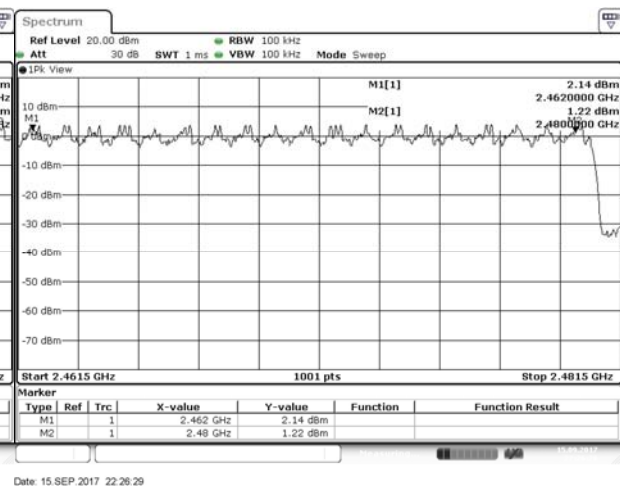
2462-2480MHz
