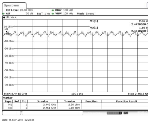
2442-2461MHz
