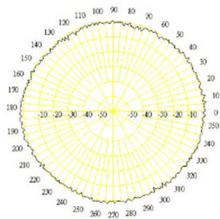
5.15~H-PLANE
