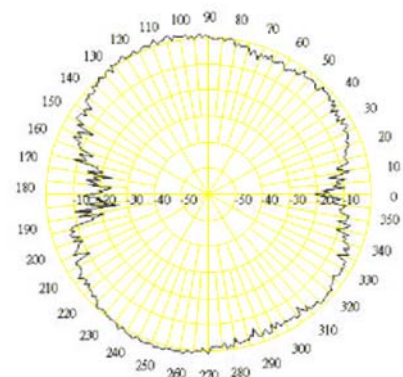
5.15~E-PLANE
