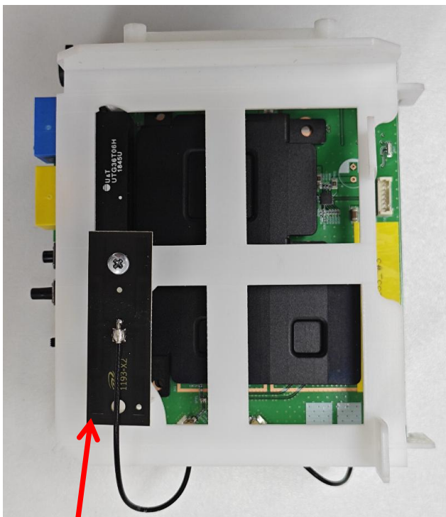
Ant1 Cable 90mm
