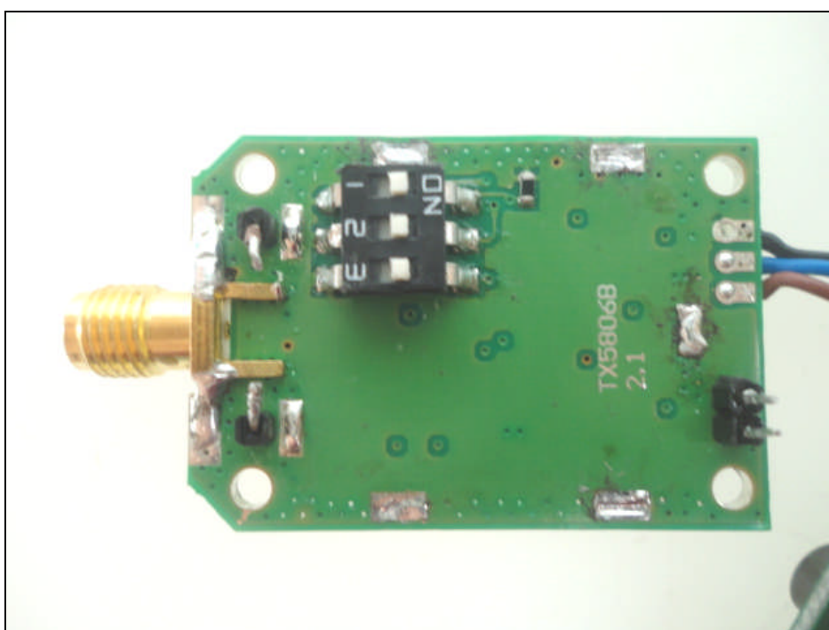
RF module
