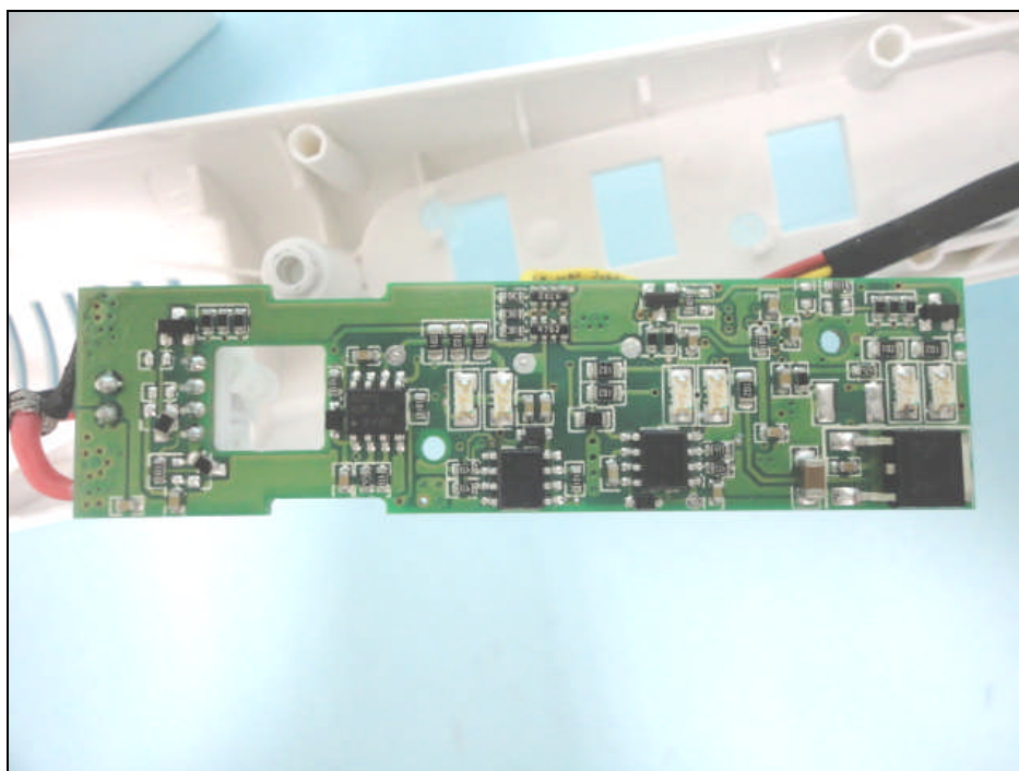
Motor Module
