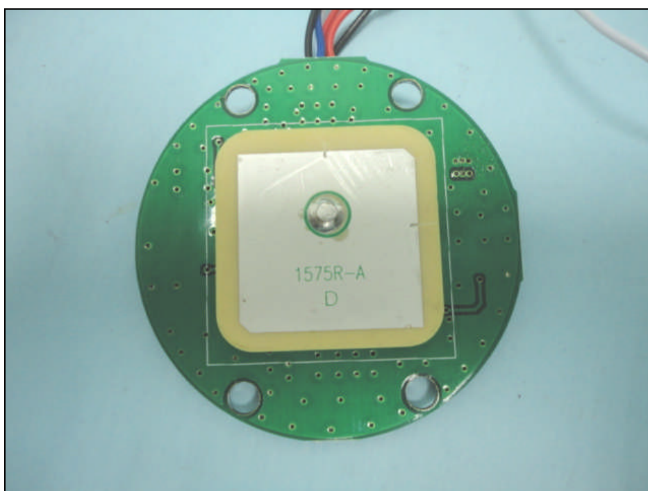
GPS Module
