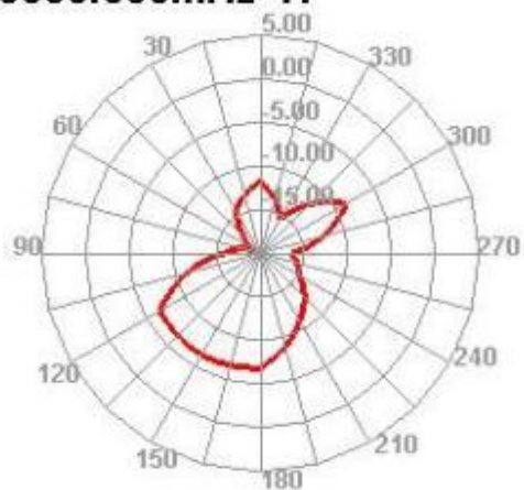
5850.000MHz H
