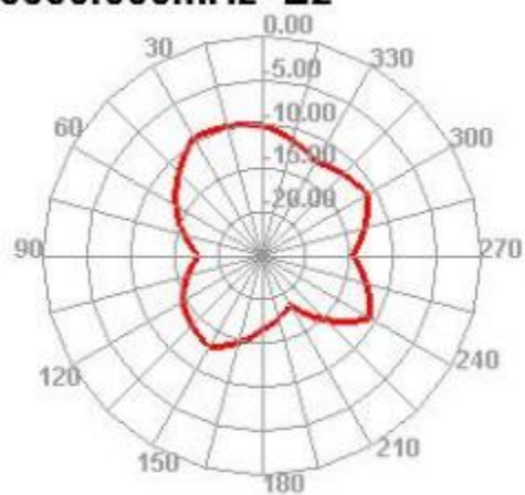
5550.000MHz E2
