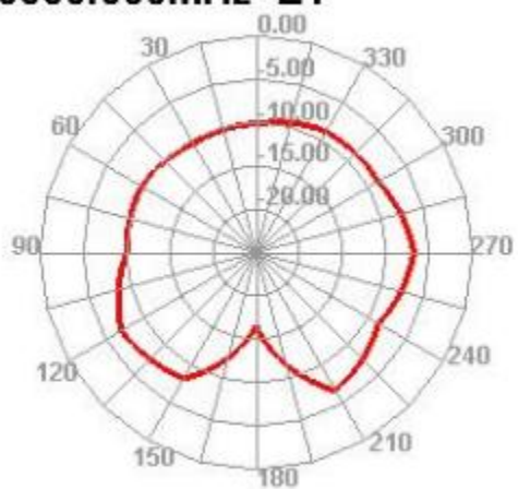
5550.000MHz E1
