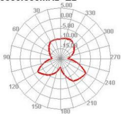
5850.000MHz E2
