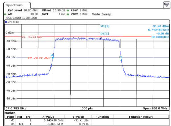
802.11ax80_6785MHz_RU_Full_ANT1 83.083MHz
