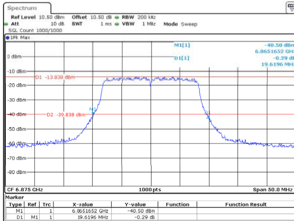
802.11a_6875MHz_ANT1 19.620MHz
