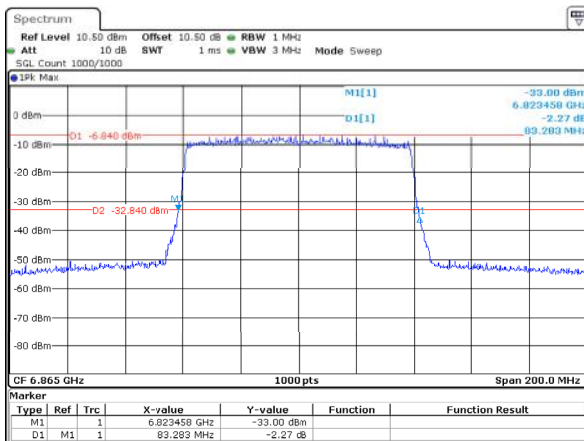
802.11ax80_6865MHz_RU_Full_ANT1 83.283MHz
