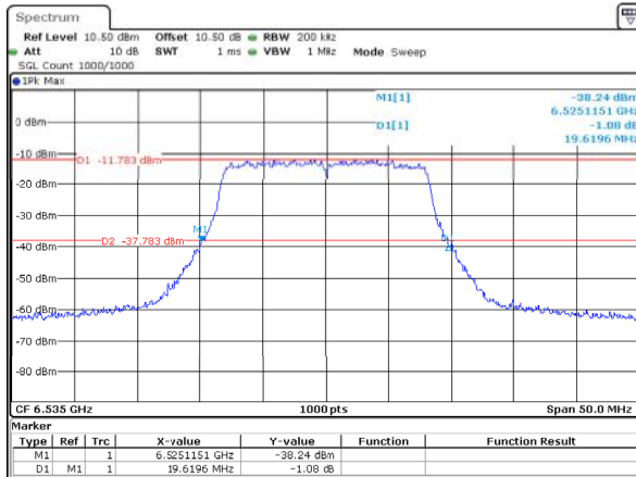
802.11a_6535MHz_ANT1 19.620MHz
