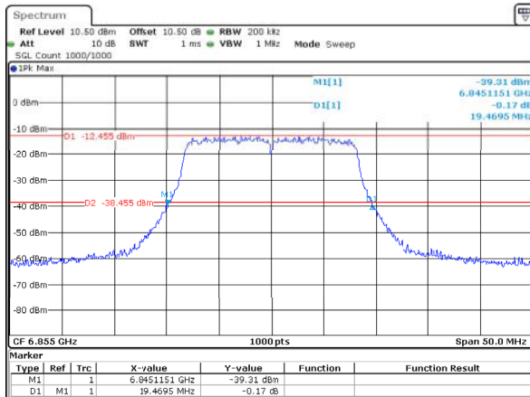
802.11a_6855MHz_ANT1 19.469MHz
