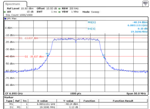
802.11a_6895MHz_ANT1 19.570MHz
