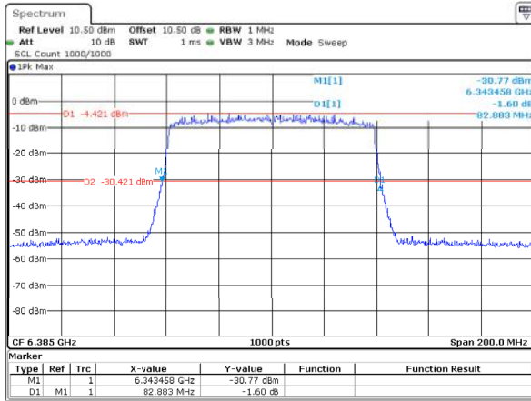
802.11ax80_6385MHz_RU_Full_ANT1 82.883MHz
