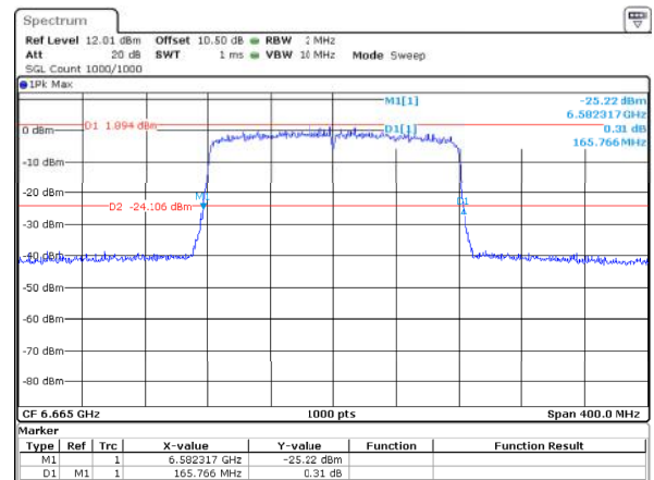
802.11ax160_6665MHz_RU_Full_ANT1 165.766MHz
