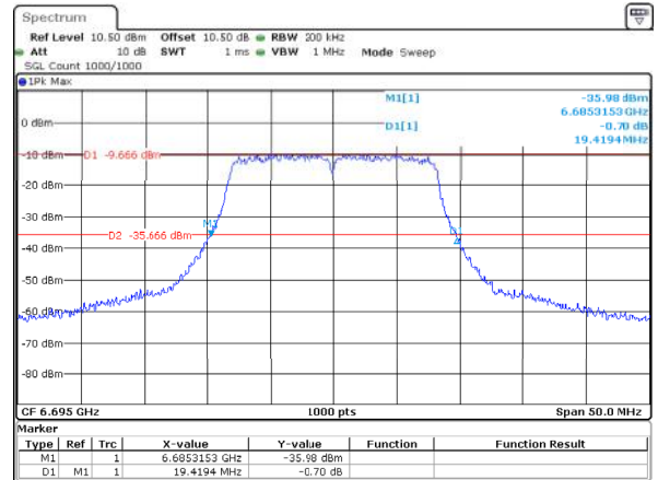
802.11a_6695MHz_ANT1 19.419MHz
