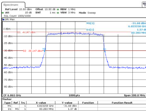
802.11ax80_6865MHz_RU_Full_ANT2 83.283MHz
