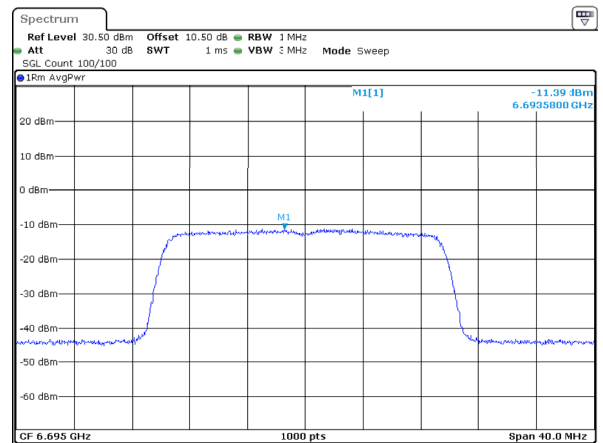
802.11ax20_6695MHz_RU_Full_ANT1 -11.39dBm/MHz
