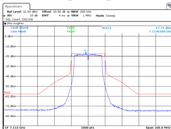
802.11a_7115MHz_ANT 2
