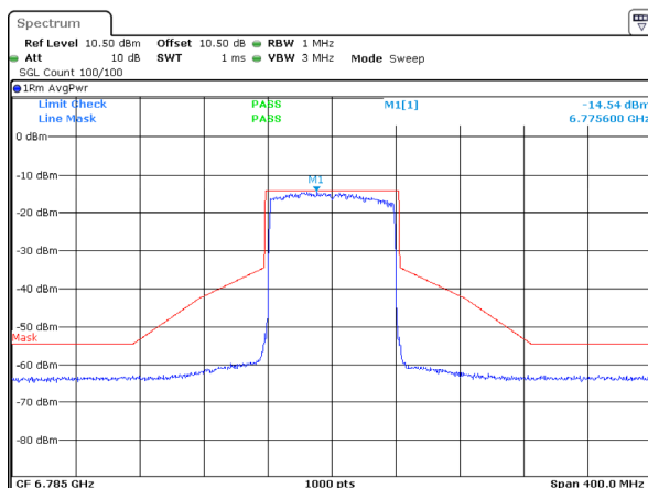
802.11ax80_6785MHz_RU_Full_ANT 1
