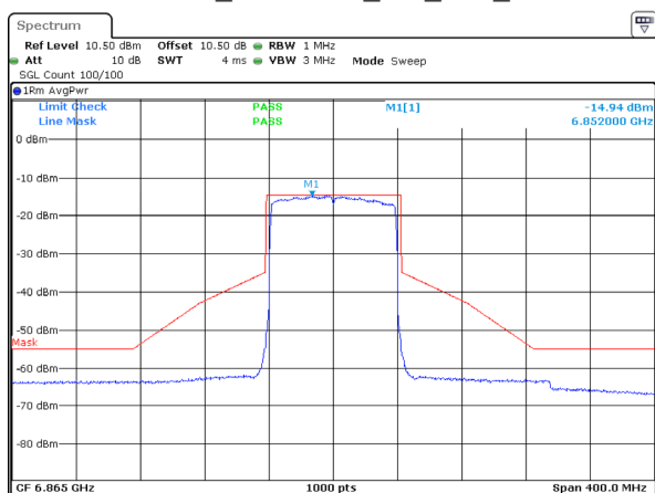
802.11ax80_6865MHz_RU_Full_ANT 2
