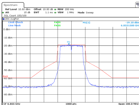
802.11a_6855MHz_ANT 2
