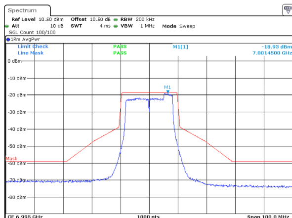
802.11a_6995MHz_ANT 1
