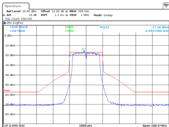
802.11a_6695MHz_ANT 2
