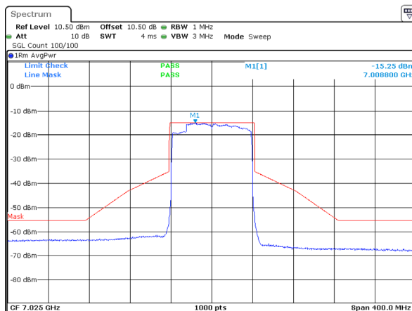
802.11ax80_7025MHz_RU_Full_ANT 1
