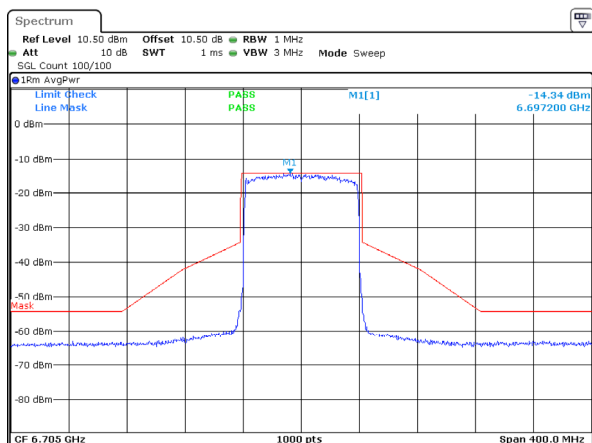
802.11ax80_6705MHz_RU_Full_ANT 1
