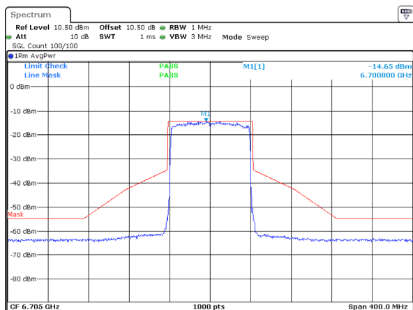
802.11ax80_6705MHz_RU_Full_ANT 2
