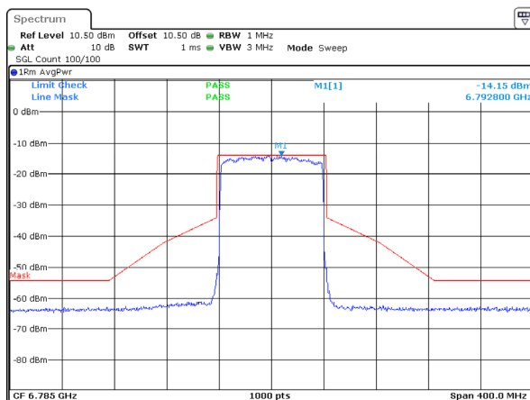
802.11ax80_6785MHz_RU_Full_ANT 2
