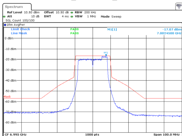
802.11a_6995MHz_ANT 2
