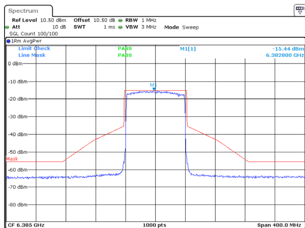
802.11ax80_6385MHz_RU_Full_ANT 1
