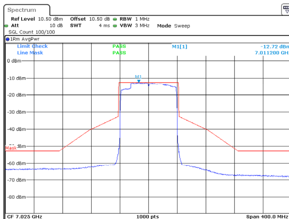
802.11ax80_7025MHz_RU_Full_ANT 2
