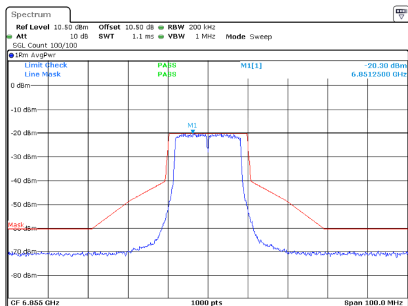
802.11a_6855MHz_ANT 1
