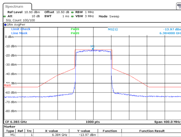
802.11ax80_6385MHz_RU_Full_ANT 2
