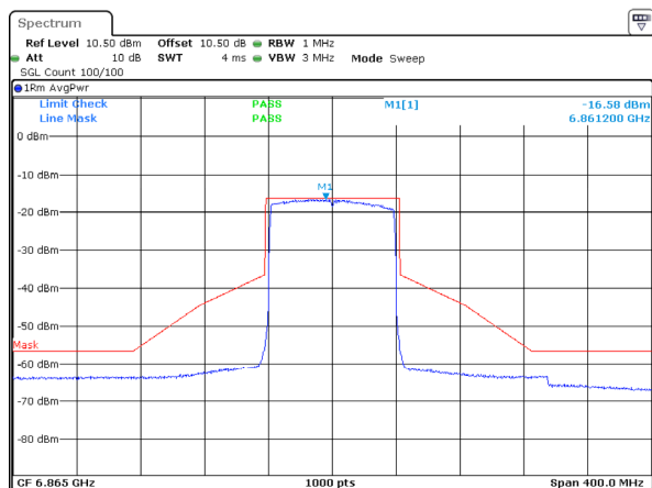
802.11ax80_6865MHz_RU_Full_ANT 1
