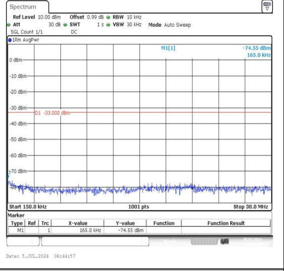
12-12-5MHz-5MHz-QPSK-QPSK-23071-23119-25
