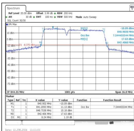
5-5-3MHz-5MHz-QPSK-QPSK-20586-20625-15R B#0-25RB#0-PASS
