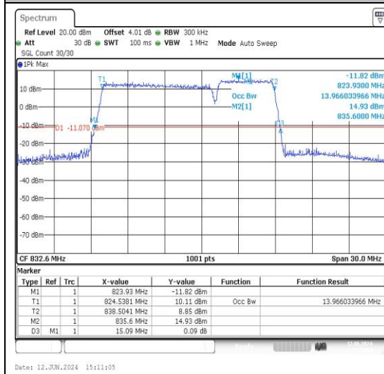
5-5-5MHz-10MHz-QPSK-QPSK-20528-20600-25 RB#0-50RB#0-PASS
