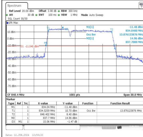
5-5-5MHz-10MHz-QPSK-QPSK-20528-20600-25 RB#0-50RB#0-PASS
