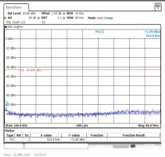
66-66-20MHz-5MHz-QPSK-QPSK-132397-132514 -1RB#99-0RB#0-0.15~30MHz-PASS
