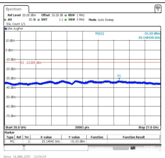
66-66-20MHz-5MHz-QPSK-QPSK-132397-132514 -1RB#0-1RB#24-20000~27000MHz-PASS
