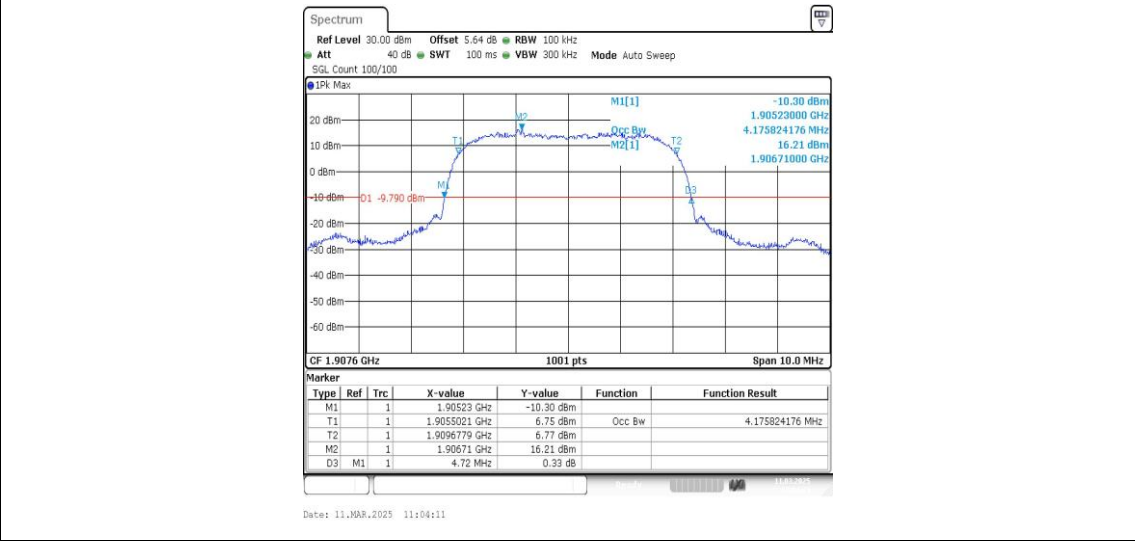
Band2-9538-3-PASS
