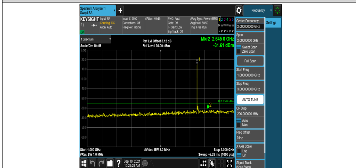
Band41-15MHz-QPSK-39725-1RB#0-Range4:1000~3000MHz
