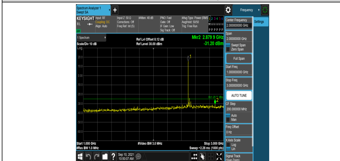
Band41-20MHz-QPSK-39750-1RB#0-Range4:1000~3000MHz
