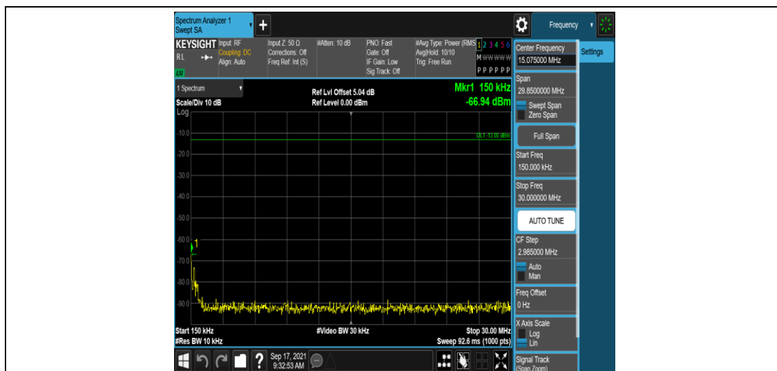
Band71-15MHz-QPSK-133197-1RB#0-Range2:0.15~30MHz
