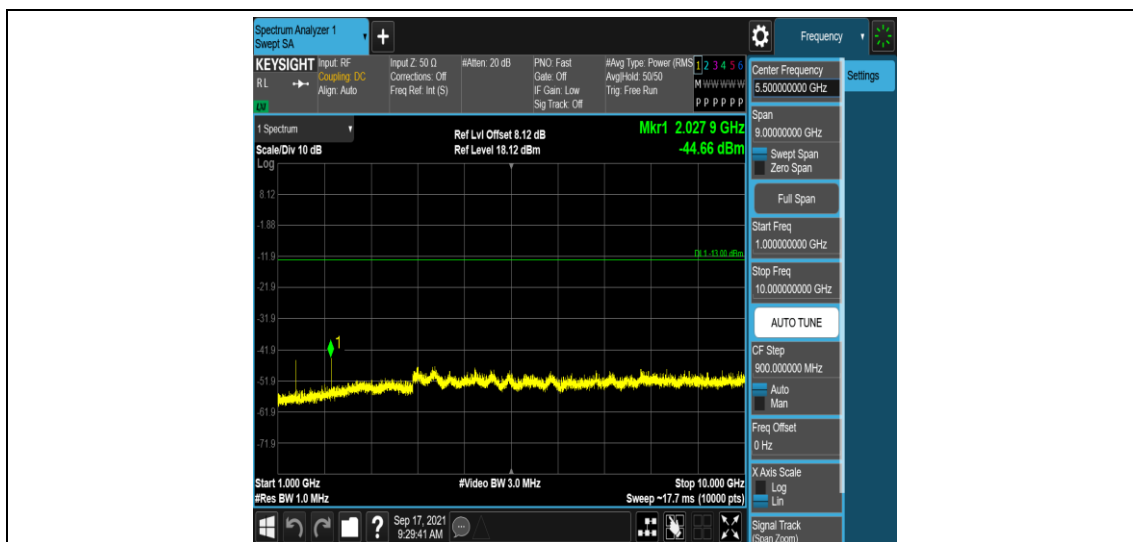
Band71-10MHz-QPSK-133297-1RB#0-Range4:1000~10000MHz
