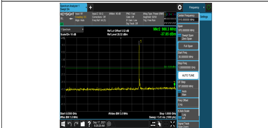
Band71-10MHz-QPSK-133297-1RB#0-Range3:30~1000MHz
