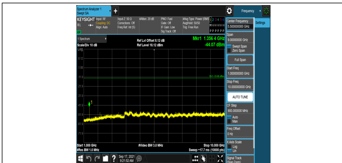
Band71-5MHz-QPSK-133297-1RB#0-Range4:1000~10000MHz
