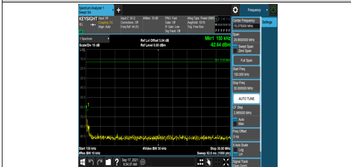
Band71-15MHz-QPSK-133297-1RB#0-Range2:0.15~30MHz
