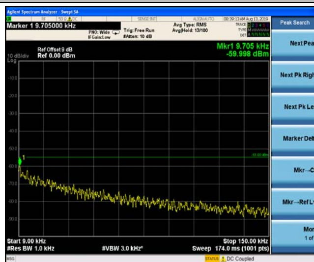
Band41_10MHz_QPSK_41540_1RB#0
