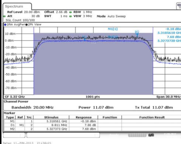
HT20 [Port 3]
