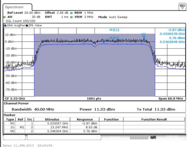
HT40 [Port 3]
