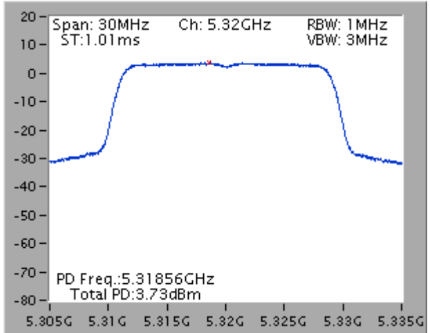
HT20
