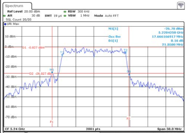
HT20
