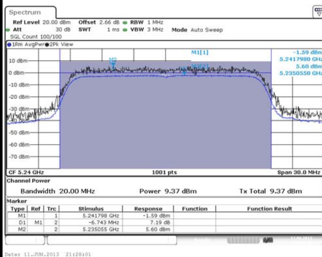
HT20 [Port 3]
