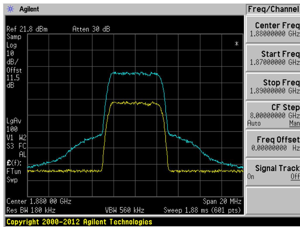
Uplink. Band 2 &amp; 25. WCDMA/LTE
