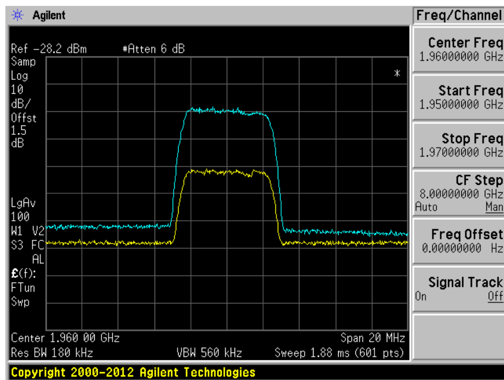
Downlink. Band 2 &amp; 25. WCDMA/LTE
